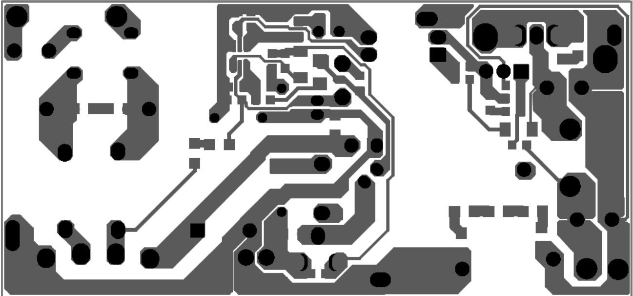
Bottom Layer
